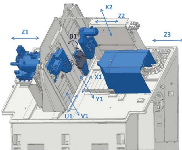
Skelet stroje K'MX 816 CLEVER s plynule řízenou B-osou
