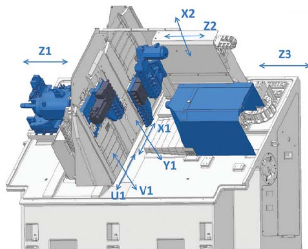
Skelet standardního stroje K'MX 816 CLEVER
